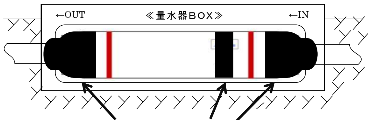
ITB設置後(P8参照)、防食テープを巻く
