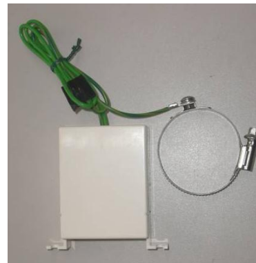
ITB (Ion Tuning Box) (コンデンサーに同梱されていません) (交換の目安は5年です)
